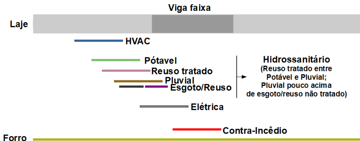
Figura 50 – Esquema 2 - Níveis de Trabalho - Entreforro – Vigas Faixas
