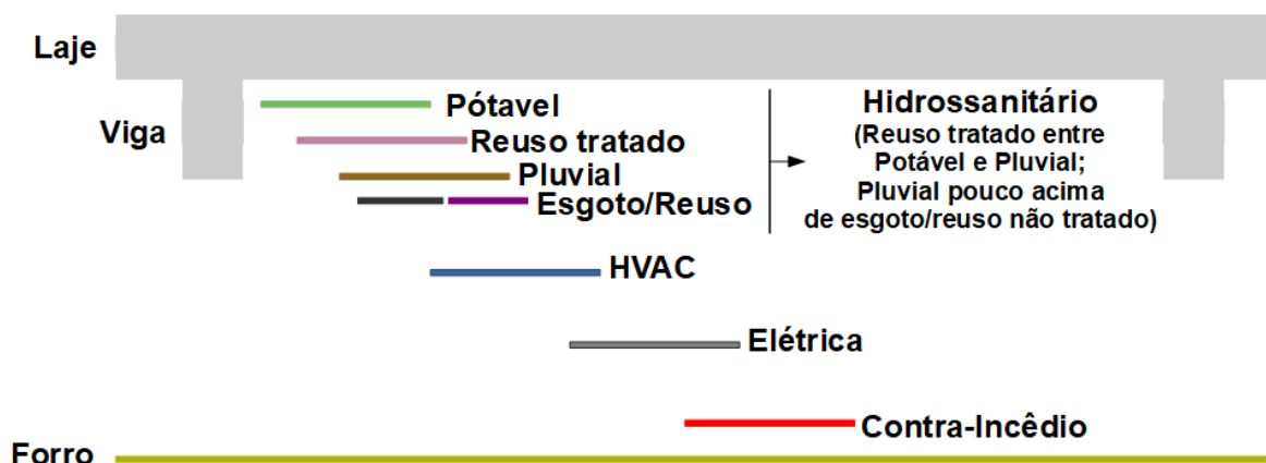
Figura 49 – Esquema 1 - Níveis de Trabalho - Entreforço – Vigas
