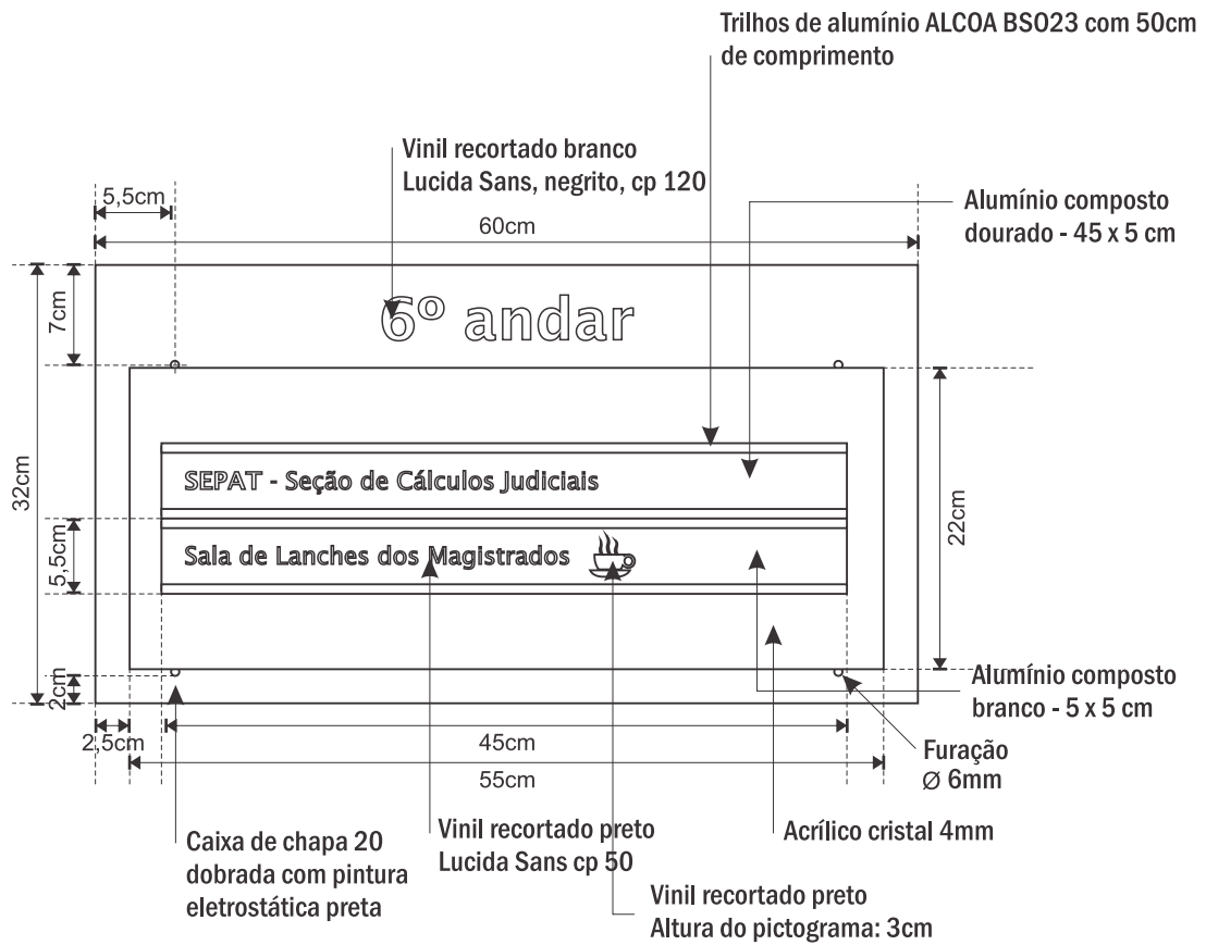
visão frontal escala 1:6
